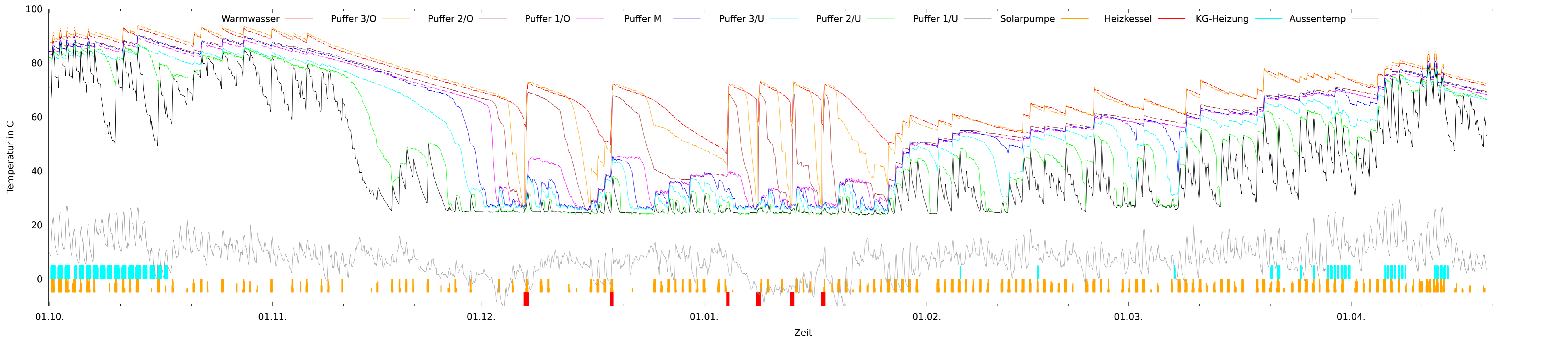
Solarwerte Winterhalbjahr 2023/2024
