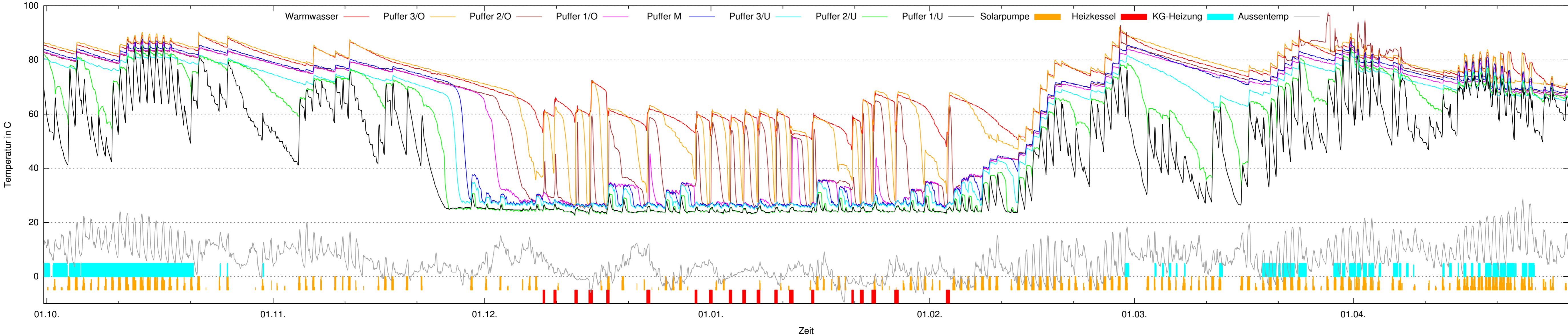
Solarwerte Winterhalbjahr 2018/2019
