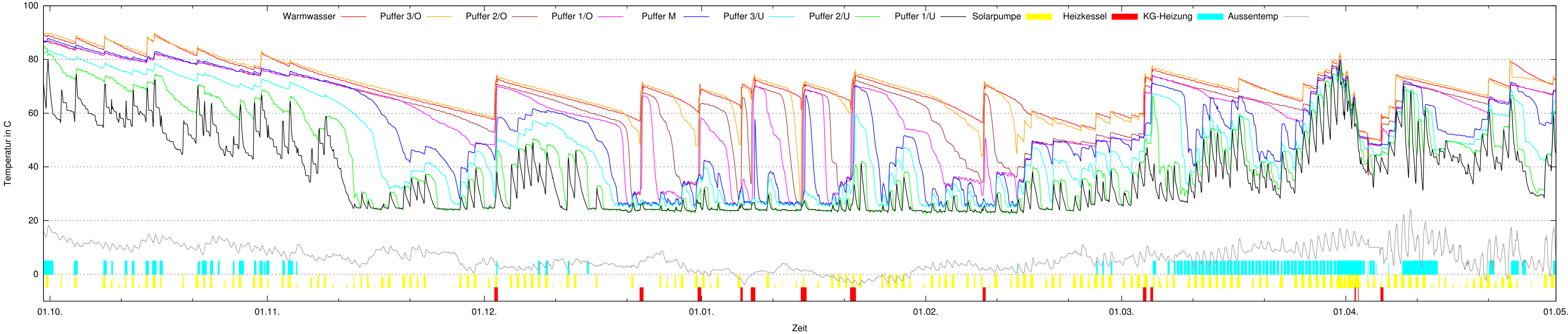
Solarwerte Winterhalbjahr 2016/2017
