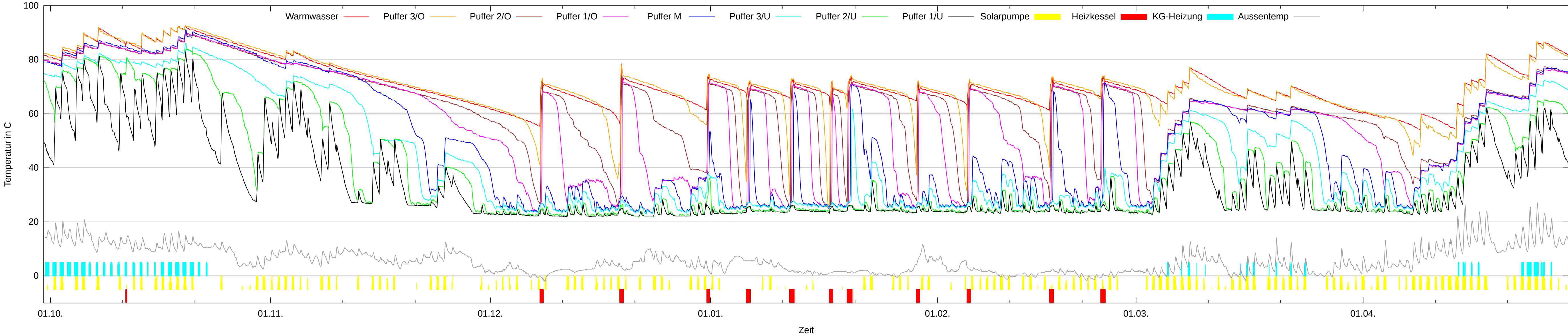
Solarwerte Winterhalbjahr 2012/13
